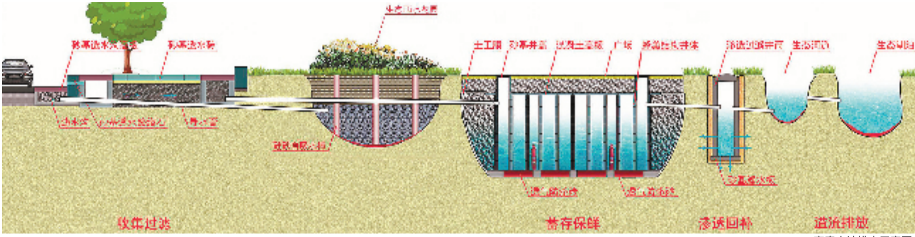
富春山馆排水示意图。
